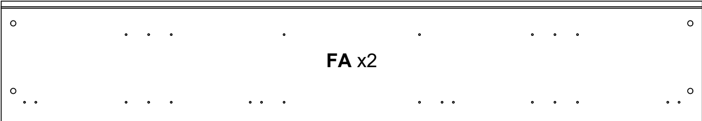
1988x342x18mm
